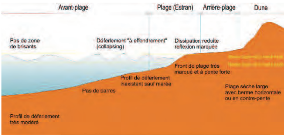
Figure 2.3 Le profil réfléchissant. © Carlos Ley
