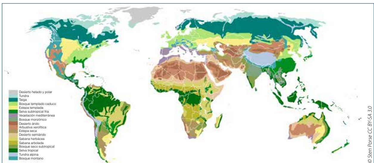
Figura 1 – Clasificación de los hábitats terrestres a una resolución de 15 ES por 1 km². Las montañas proveen numerosos servicios ecosistémicos (Grêt-Regamey et al. 2012).
